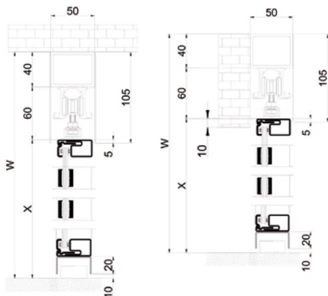
Deckenmontage
